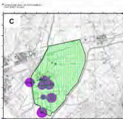
Figura 19: Distribuzione territoriale di [Mn] in base ai range di concentrazione. A: [Mn] < 250ppb; B: 250ppb < [As] < 3000ppb; C: [As] > 3000ppb. L'area evidenziata in verde è quella che delimita il Perimetro .
